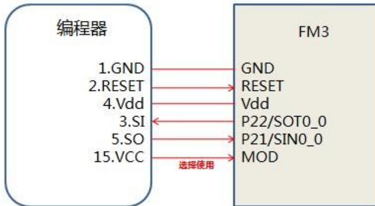
图 5：FM3 系列链接示例
