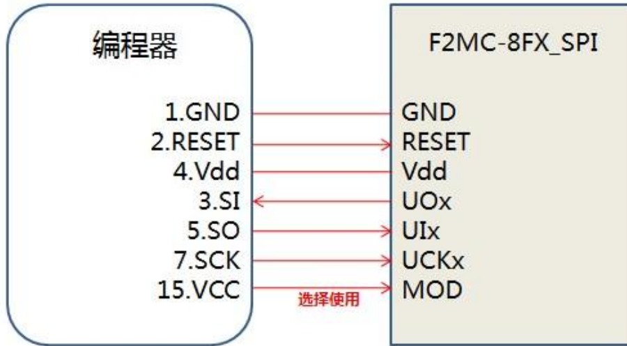
图 2: F2MC-8FX_SPI 连接示例
