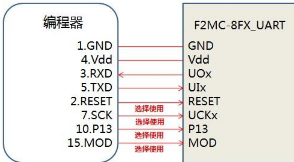
图 3: F2MC-8FX_串口连接示例
