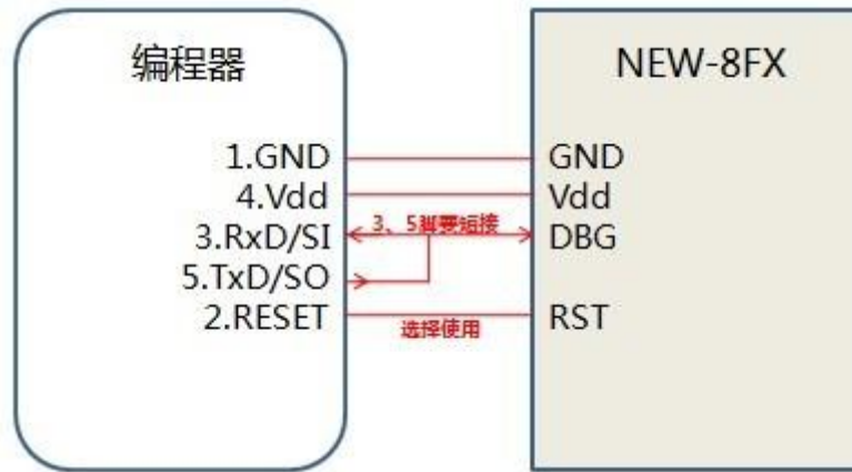
图 4：NEW-8XF 系列链接示例
