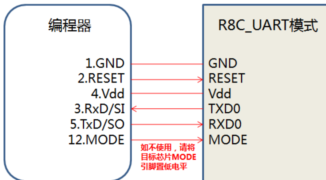
图 7：R8C 系列 UART 模式连接示例
